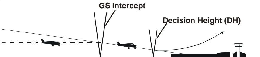
Fig. 3-15. Straight-In ILS Approach
